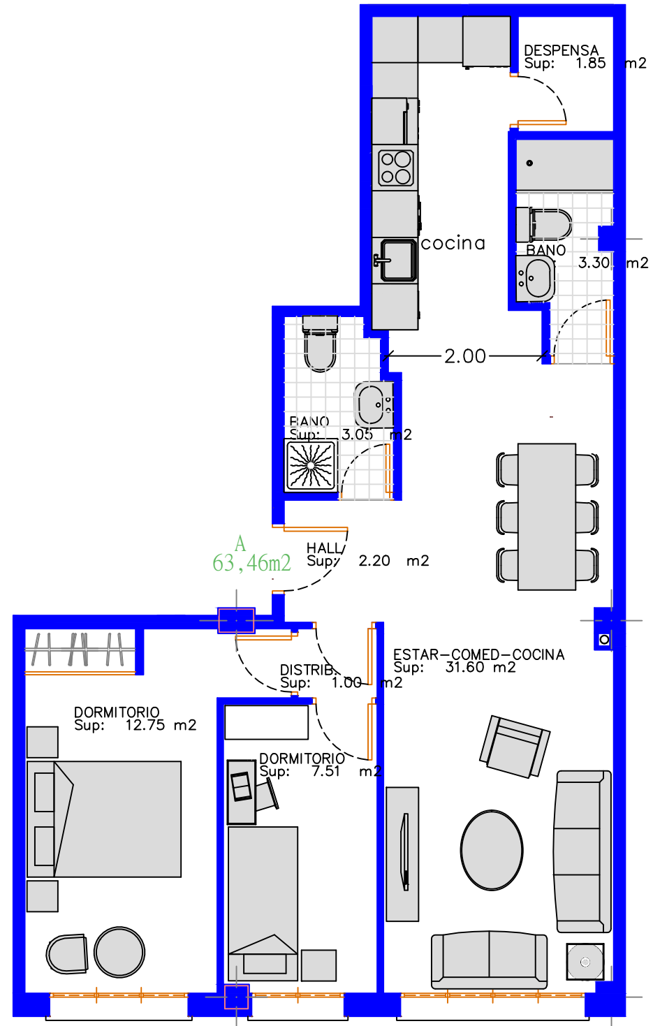
Planta Baja
