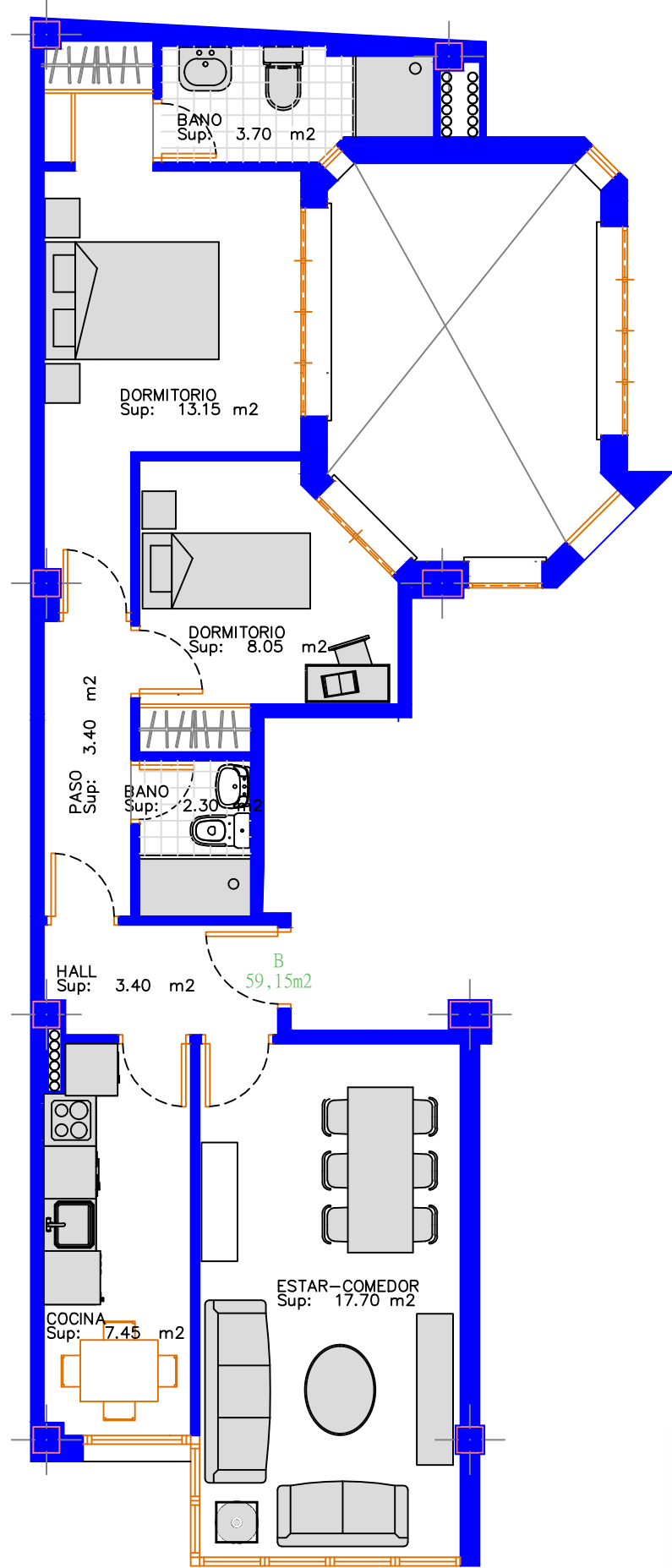
Planta Tipo (2ª y 3ª)
